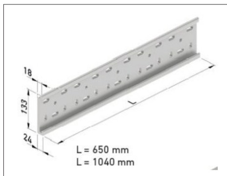
Konsola ścienna 650 / 1040 mm
