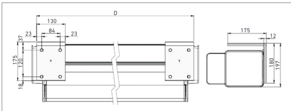
Wspornik sufitowy do konsoli ściennej. D - rozstaw konsol.
