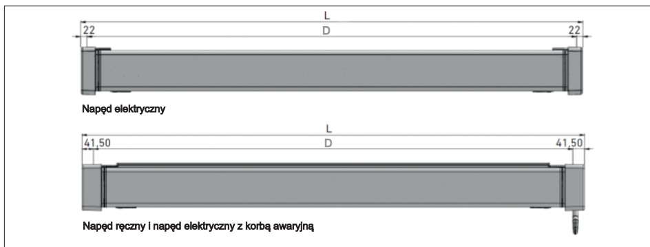
Rozstaw konsol montażowych D. L - szerokość całkowita.
