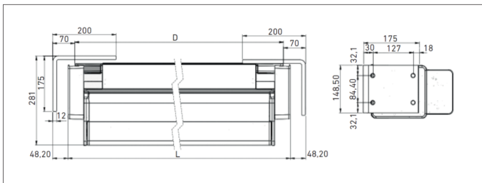
Wspornik wewnętrzny do konsoli ściennej. D - rozstaw konsol.
