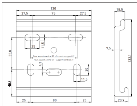
Konsola ścienna 130 mm
