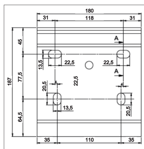
Konsola montażowa 180 mm
