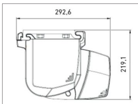
Montaż sufitowy
