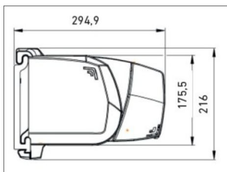
Montaż ścienny
