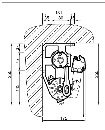
Basic-Plus - widok od strony przekładni. Montaż uniwersalny ścienny lub sufitowy.
