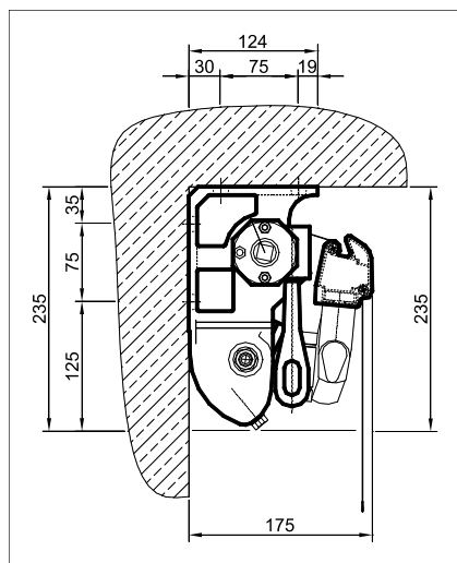
Basic - widok z boku od strony przekładni. Montaż uniwersalny ścienny lub sufitowy.
