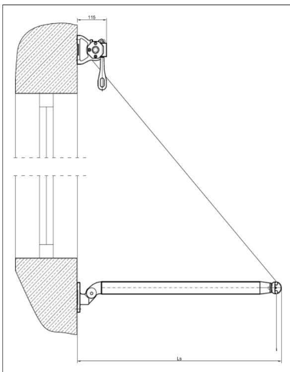
Egadi - markiza rozwinięta do kąta prostego
