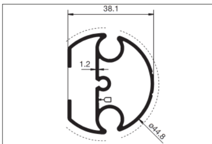
Profil dolny do systemu bez prowadzenia linkowego
