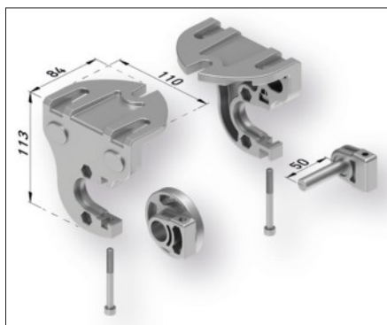
Wspornik montażowy rury - standardowy
