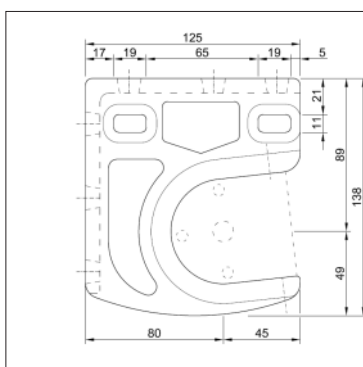
Wspornik montażowy rury - powiększony
