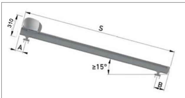
Montaż do podkonstrukcji - kaseta standardowo z tyłu
