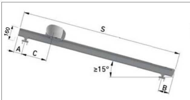
Montaż do podkonstrukcji - kaseta cofnięta
