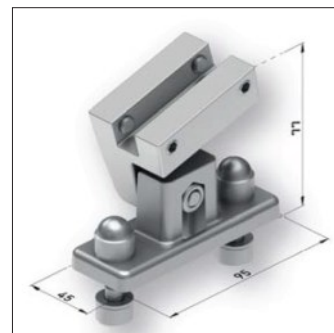
Wspornik montażowy prowadnicy z regulacją kąta nachylenia.
