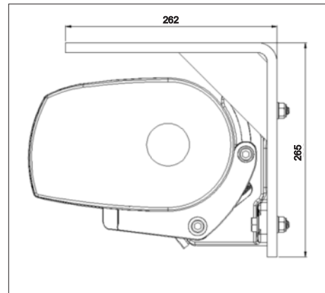
Montaż sufitowy - 15° - silnik
