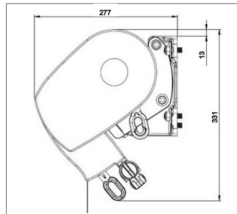
Montaż ścienny - 50° - falbana zwijana
