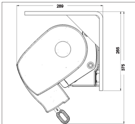
Montaż sufitowy - 50° - falbana zwijana
