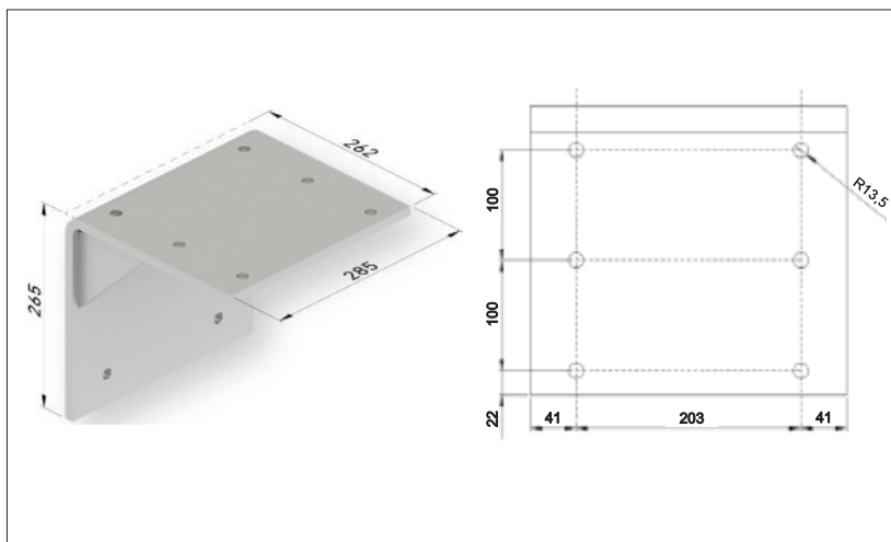
Wspornik sufitowy do konsoli ściennej
