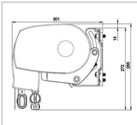
Montaż ścienny - 15° - falbana zwijana
