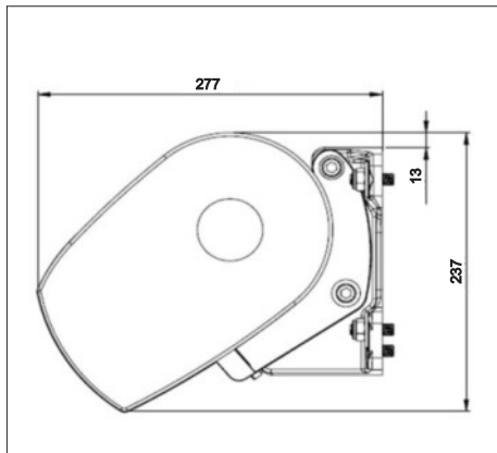
Montaż ścienny - 50° - silnik
