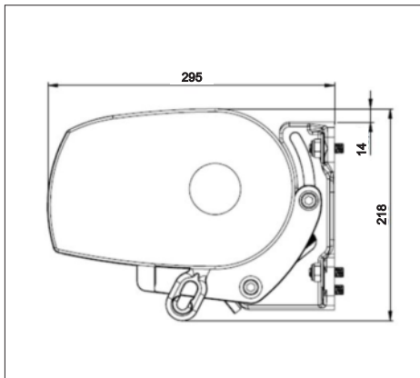
Montaż ścienny - 15° - przekładnia
