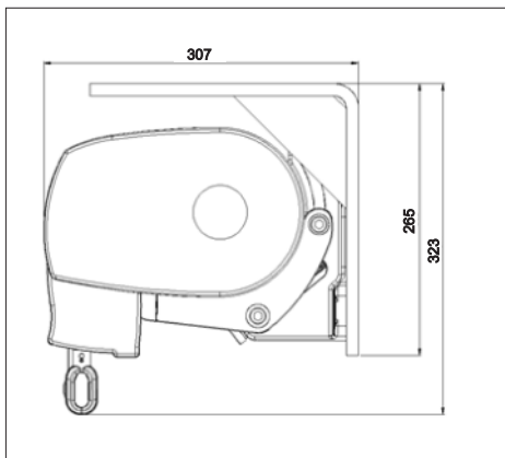
Montaż sufitowy - 15° - falbana zwijana
