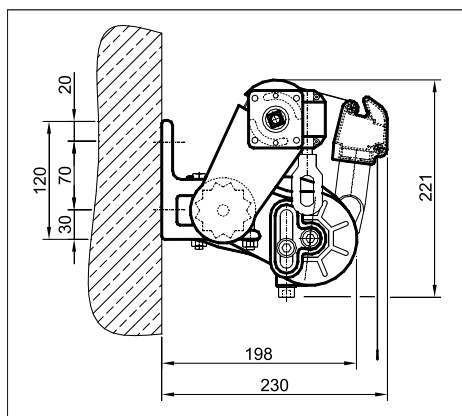
Linea - montaż ścienny
