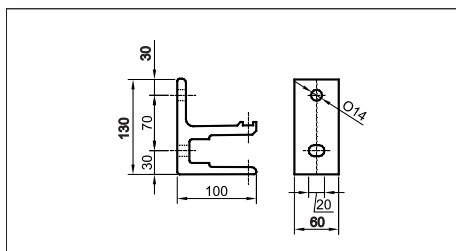
Linea-Box, Linea Wspornik montażowy ścienny
