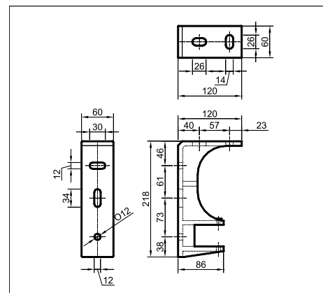
Linea-Box, Linea Wspornik montażowy ścienno-sufitowy
