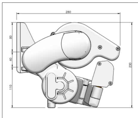
Linea-Box - montaż ścienny
