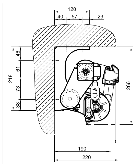
Linea - montaż uniwersalny na wspornikach ścienno - sufitowych.
