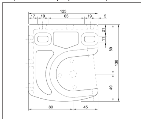
Wspornik montażowy rury - powiększony
