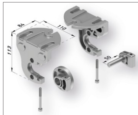
Wspornik montażowy rury - standardowy
