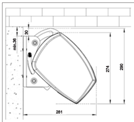
MAXIMUS - montaż ścienny - 45°
