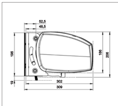
MAXIMUS - montaż ścienny - 10°
