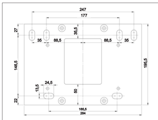
Konsola ścienna główna
