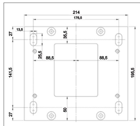
Konsola ścienna dodatkowa
