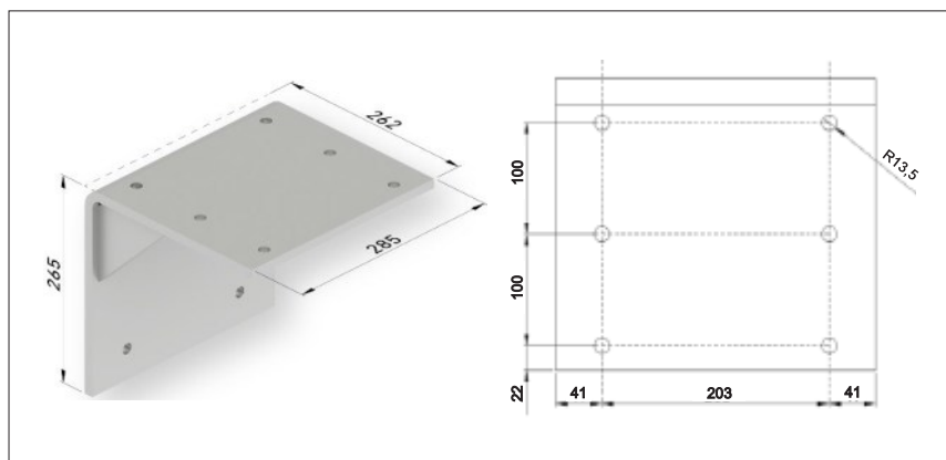
Wspornik sufitowy do konsol ściennych
