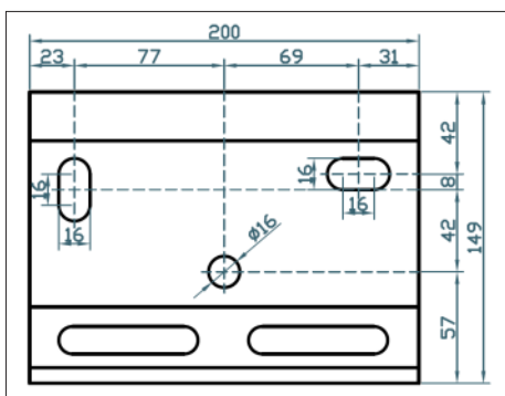
Konsola montażowa 200 mm
