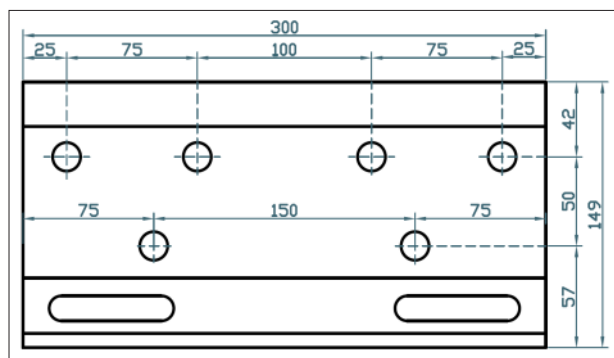
Konsola montażowa 300 mm
