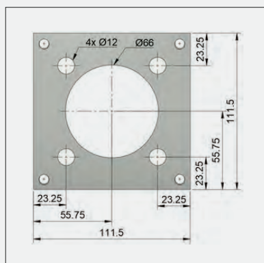
Stopa słupa wewnętrzna
