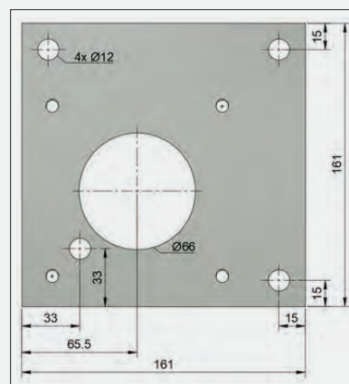
Stopa słupa narożna
