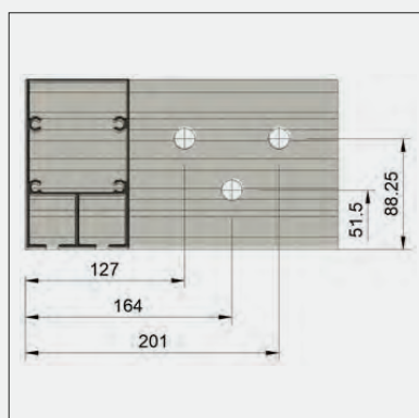
Mocowanie ściennie ramy
