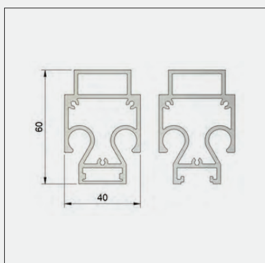
Profil wiatrowy / profil wiatrowy LED
