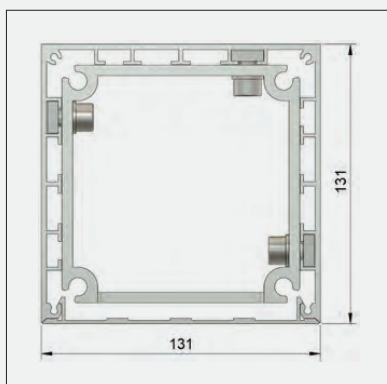
Słup + pokrywa + wzmocnienie
