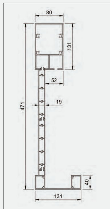
Prowadnica z rynną
