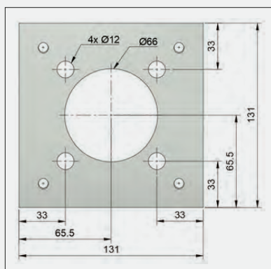
Stopa słupa zlicowana
