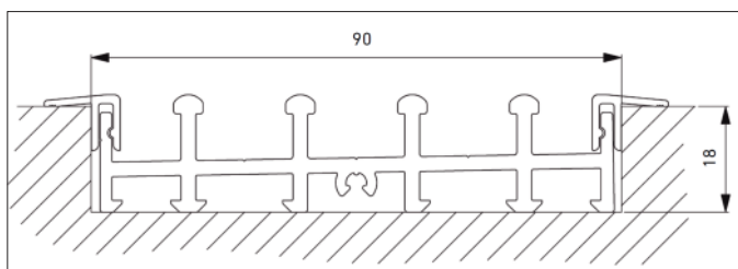
Montaż wpuszczany szyny dolnej z maskownicami (szyna dolna 4-torowa)
