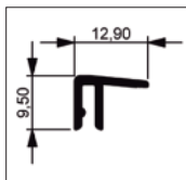
Maskownica szyny dolnej montaż wpuszczany
