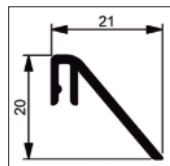
Maskownica szyny dolnej montaż nawierzchniowy
