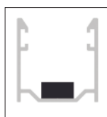
Profil boczny „U” 26x26 mm
