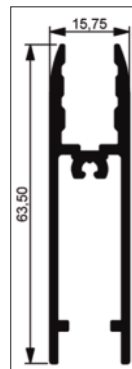
Profil dolny szyby
