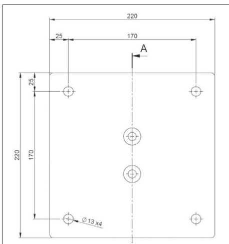
Stopa podłogowa słupa 220x220 mm, centralna
