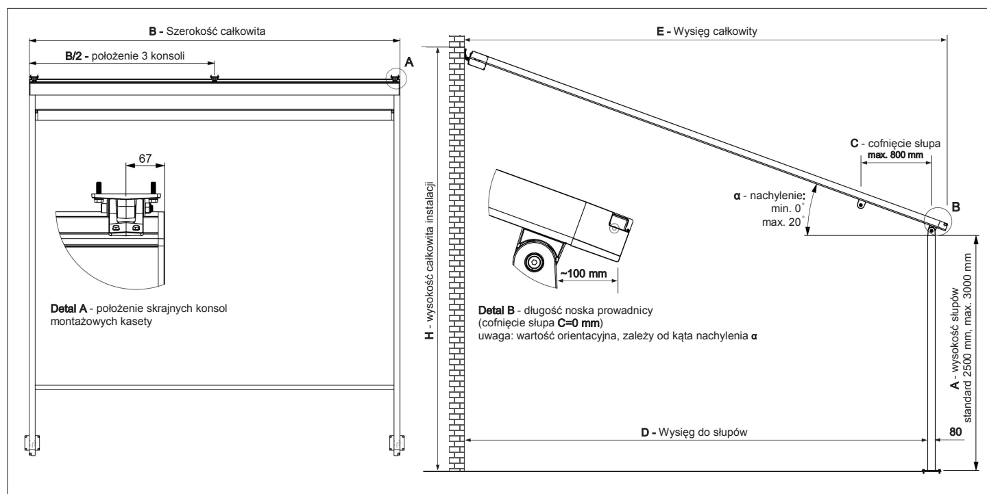
Schemat montażowy
