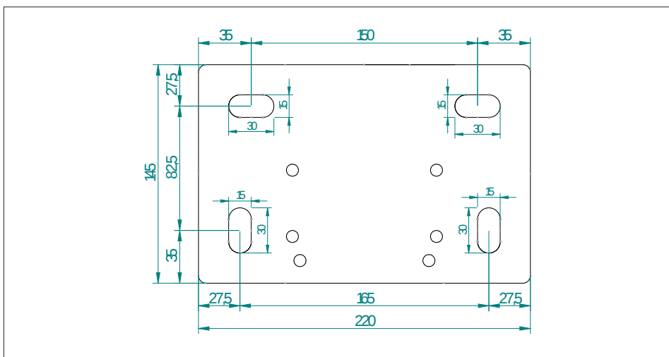
Płyta montażowa pośrednia do konsoli ściennej i sufitowej kasety - stosować do ścian z ociepleniem
