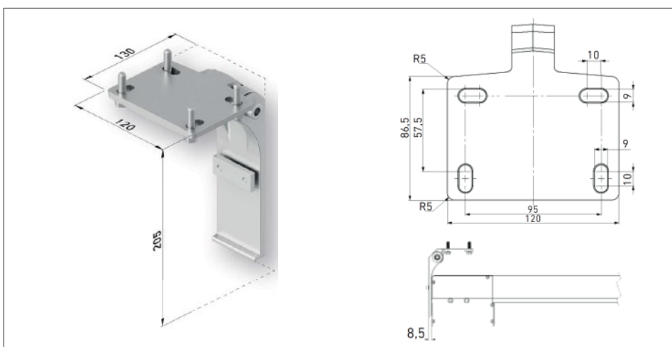
Konsola sufitowa kasety
