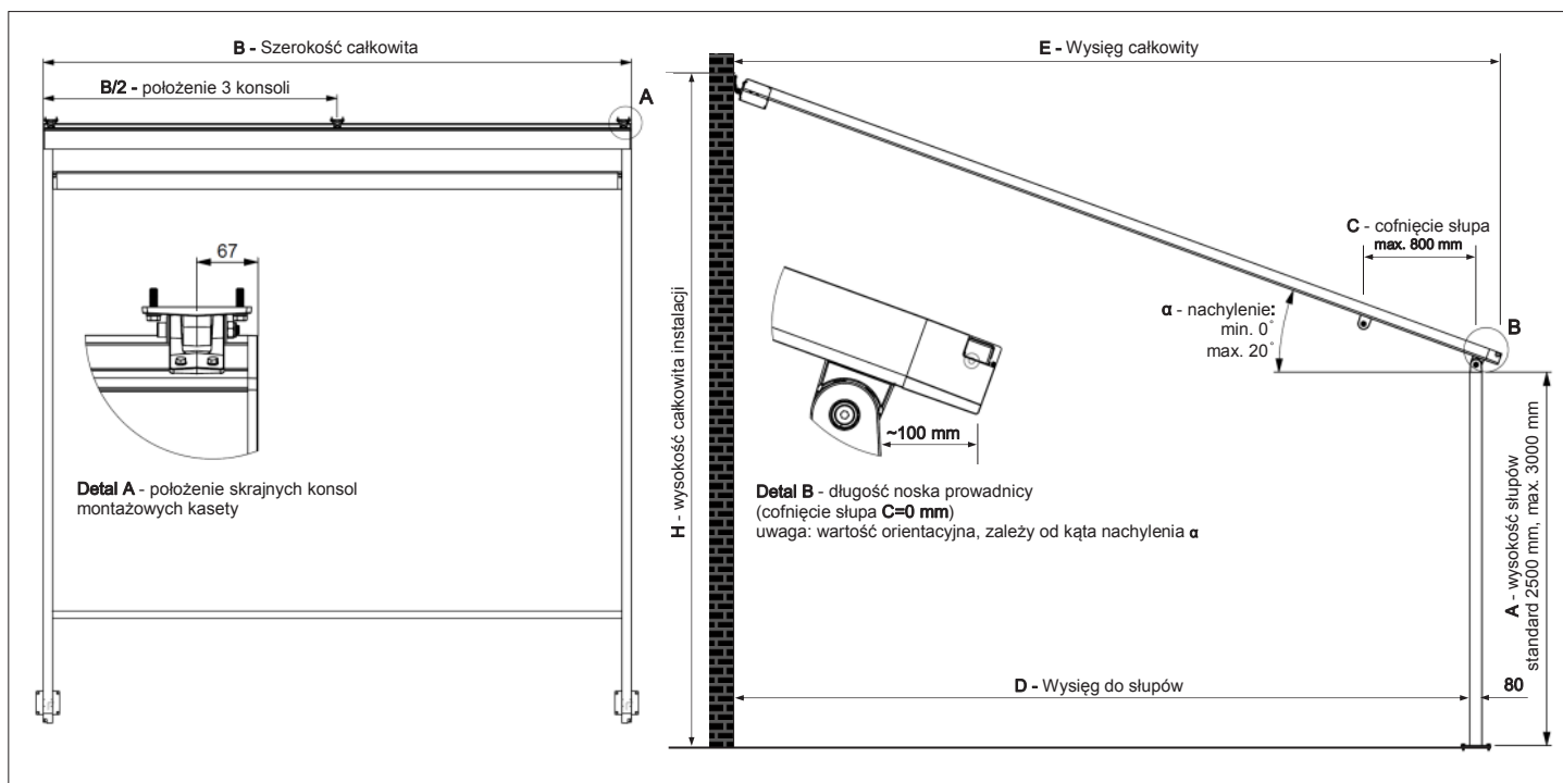
Schemat montażowy
