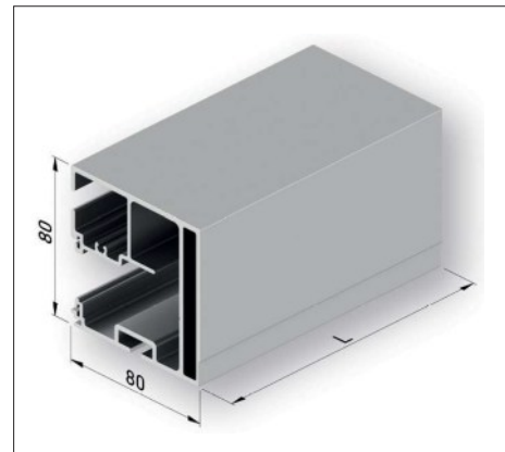
Przekrój prowadnicy
