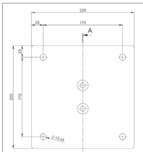
Stopa podłogowa słupa 220x220 mm, centralna
