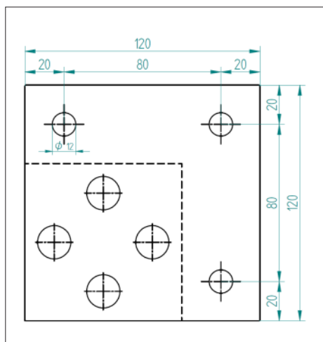
Stopa podłogowa słupa 120x120 mm, narożna
