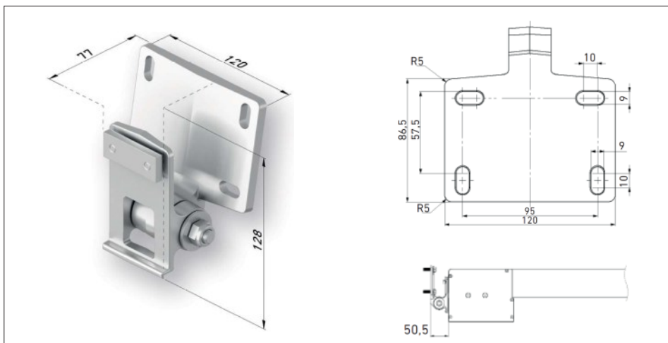
Konsola ścienna kasety
